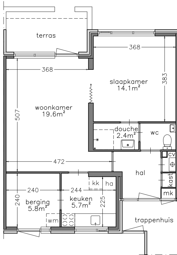
begane grond woningtype A
