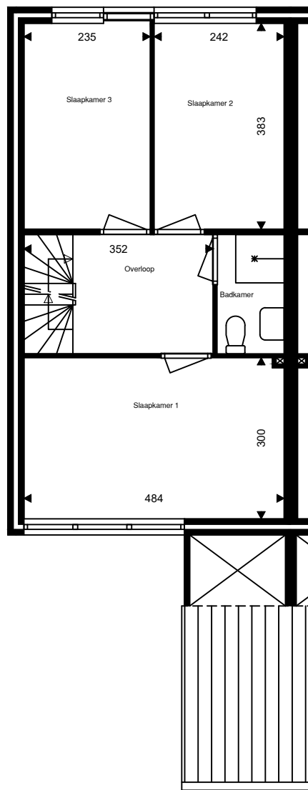
1e verdieping
