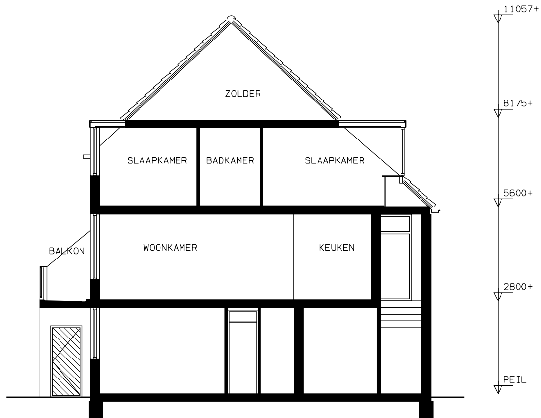
DOORSNEDE
