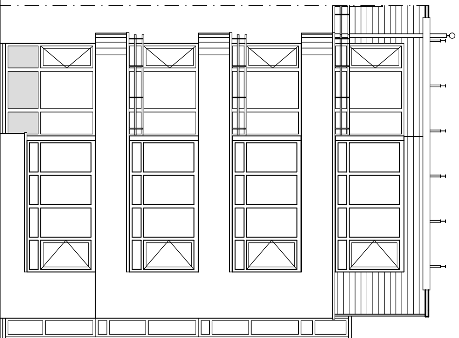
Voorgevel
