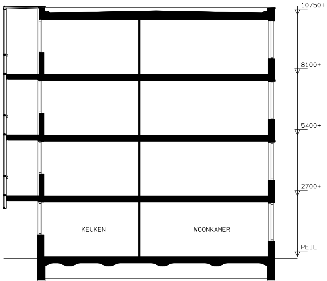
DOORSNEDE
