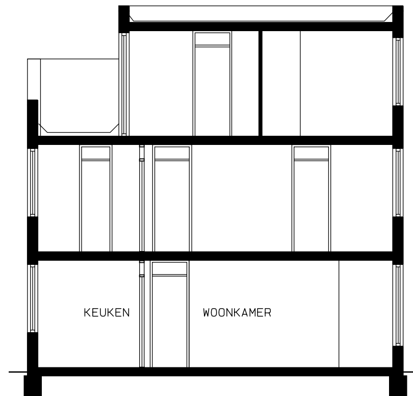
DOORSNEDE
