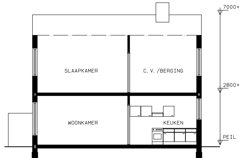
DOORSNEDE
