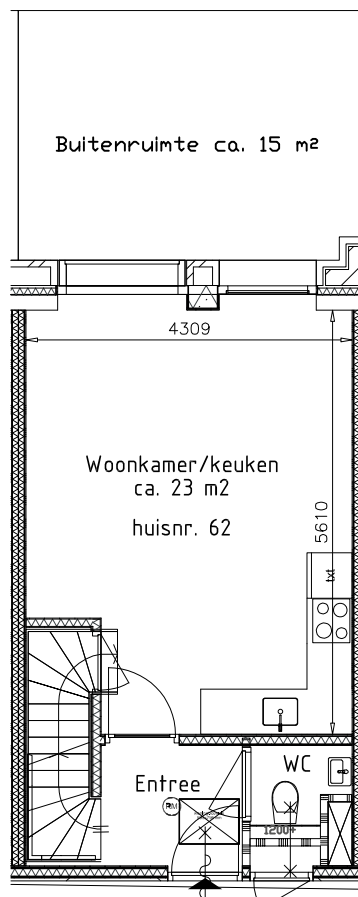
Begane grond
