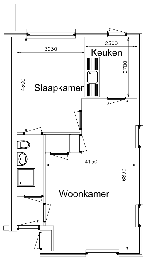
Begane grond
