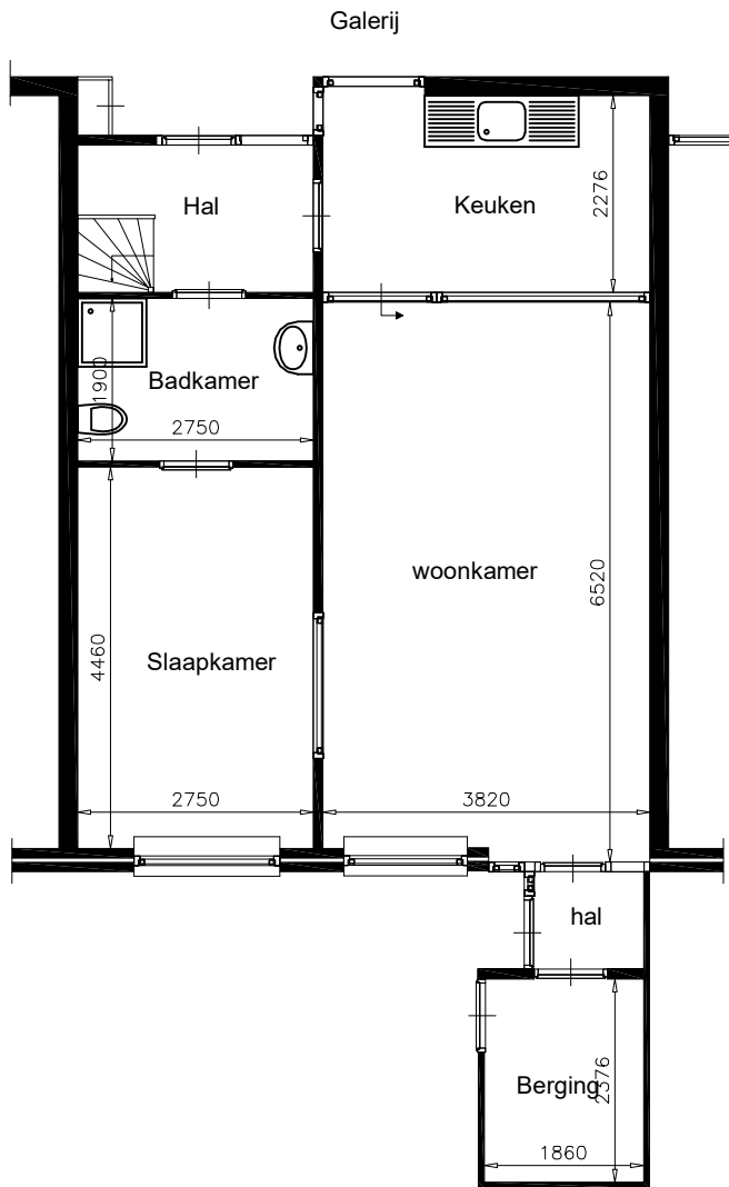
begane grond
