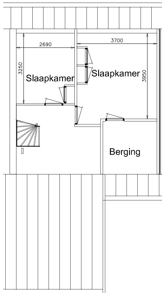
2e verdieping
