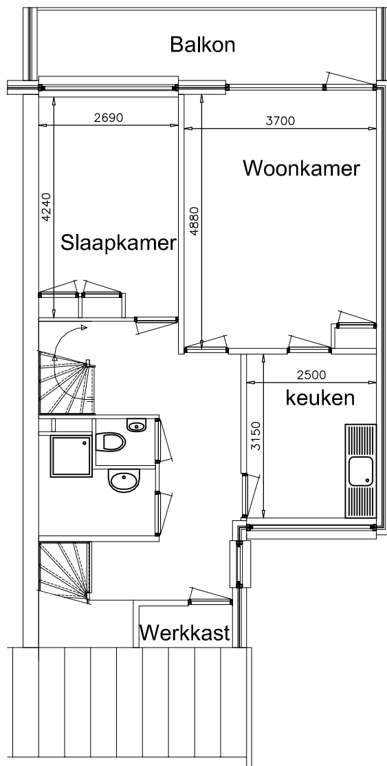
1e verdieping
