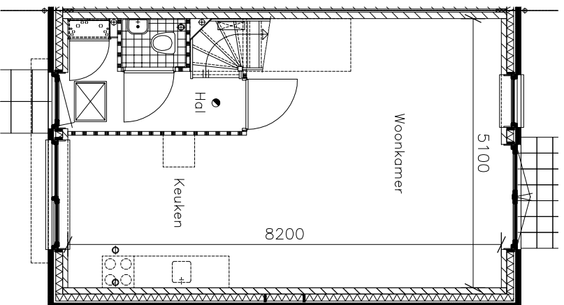
Begane grond
