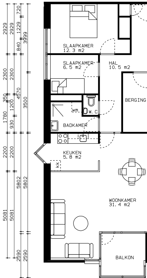
2e VERDIEPING
