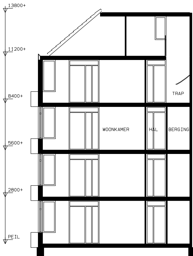
DOORSNEDE
