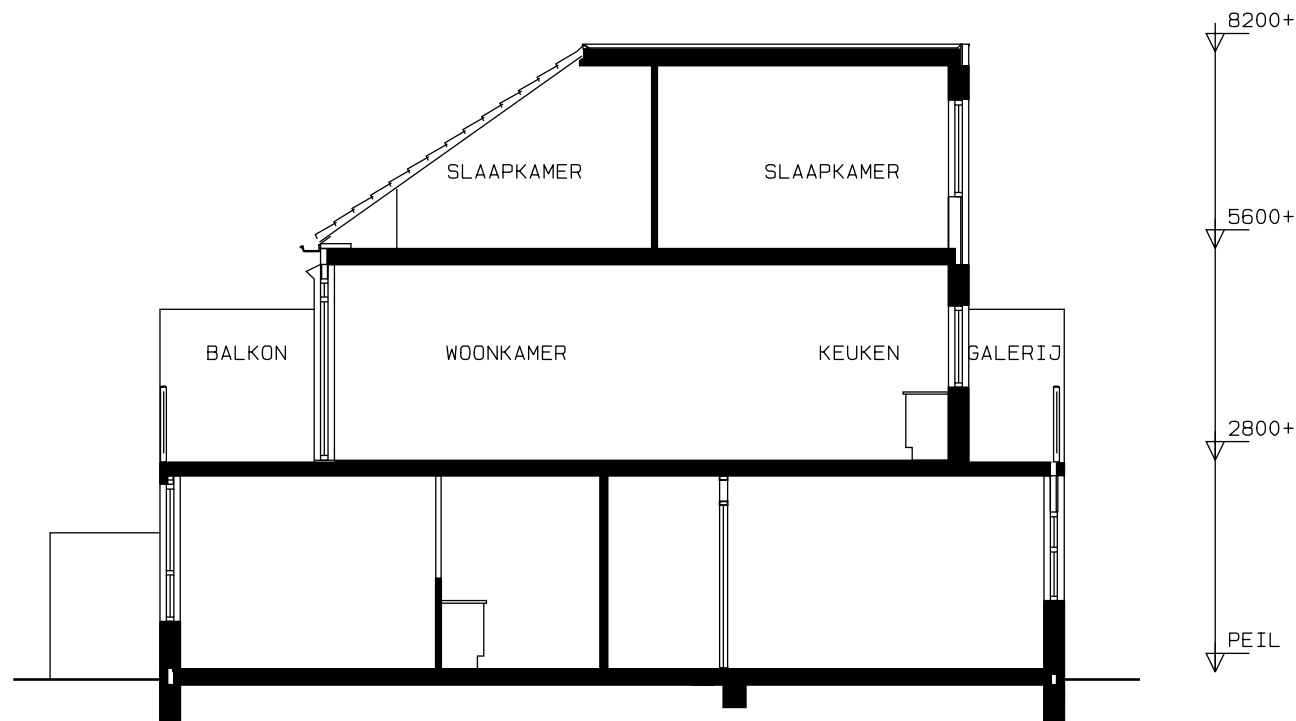
DOORSNEDE
