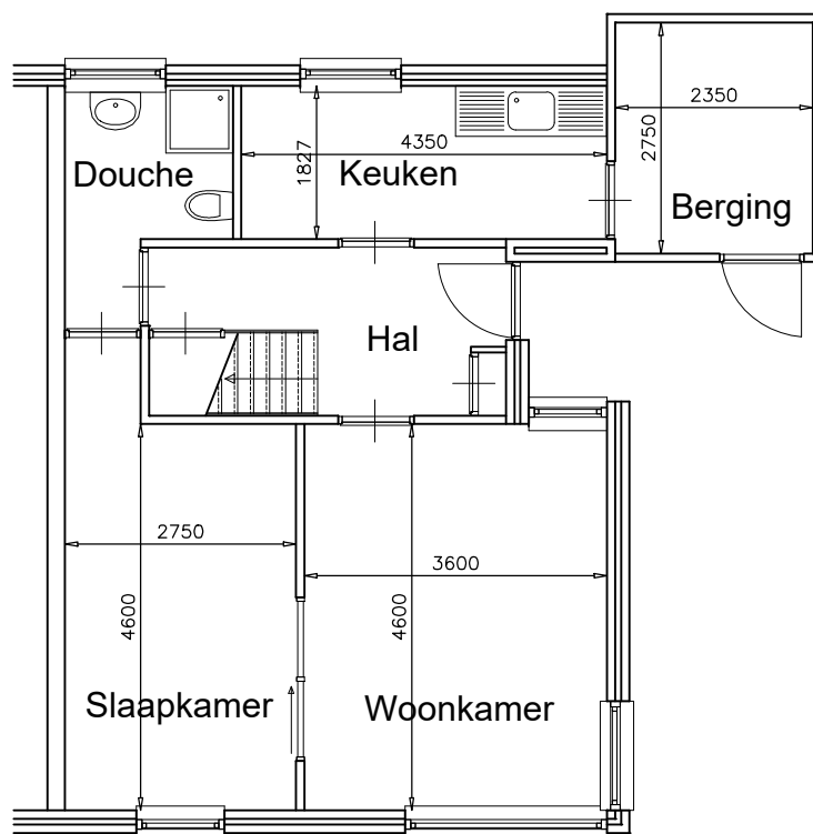
Begane grond
