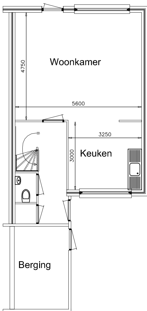
Begane grond
