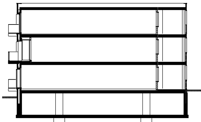
DWARSDOORSNEDE (2 HOOG)
