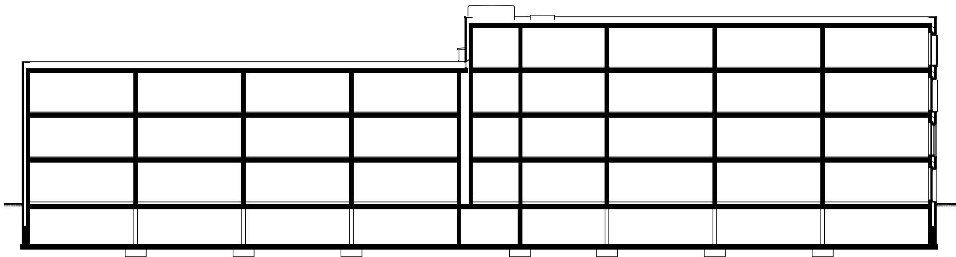
LANGSSDOORSNEDE
