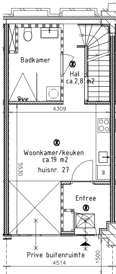
Begane grond
