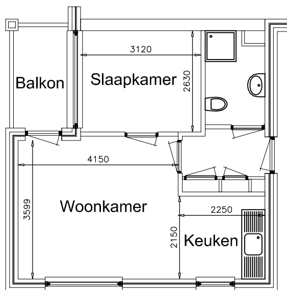
2e verdieping
