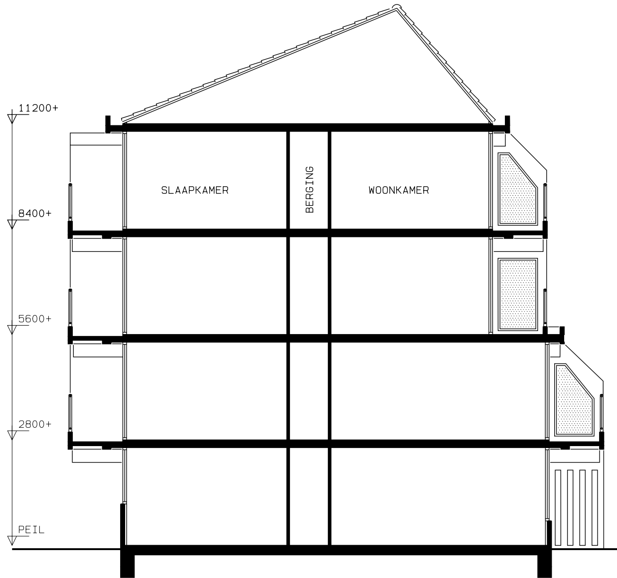
DOORSNEDE
