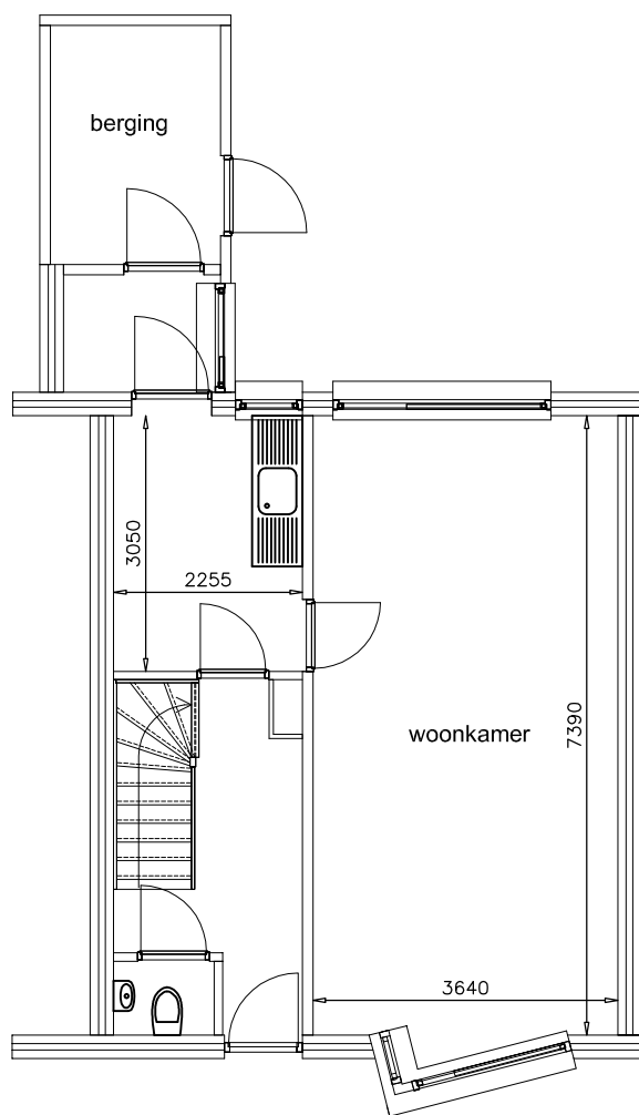
begane grond
