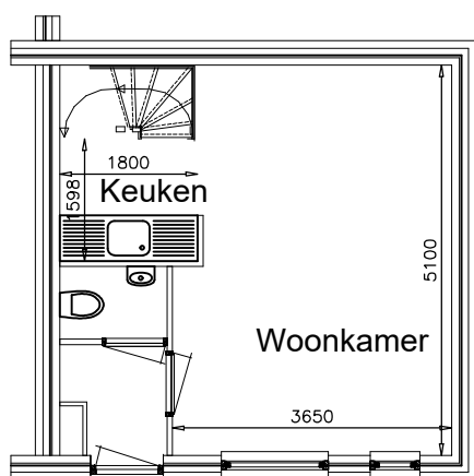
Beganegrond
