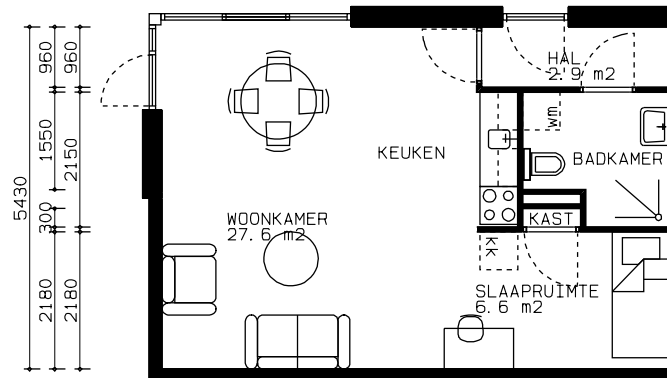
BEGANE GROND
