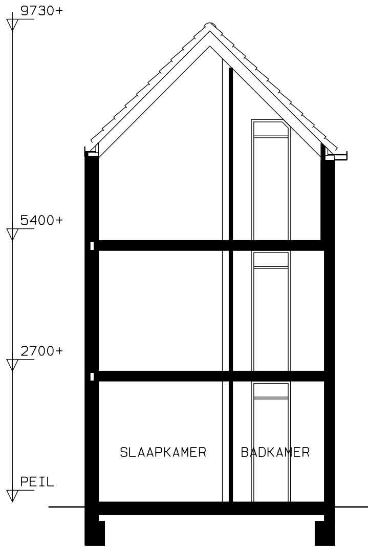
DOORSNEDE
