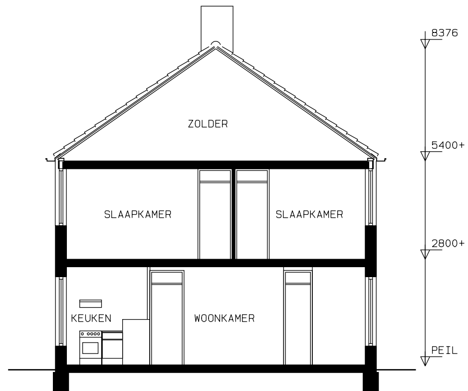
DOORSNEDE
