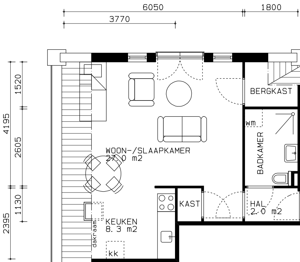
2e VERDIEPING
