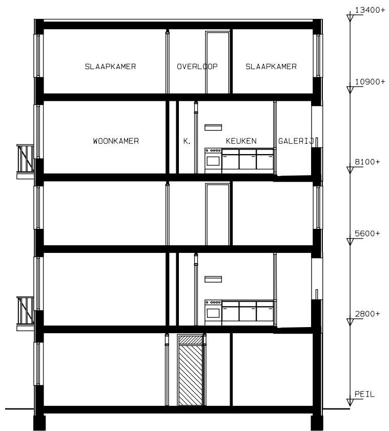
DOORSNEDE
