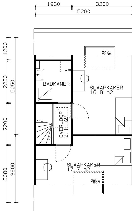
1e VERDIEPING
