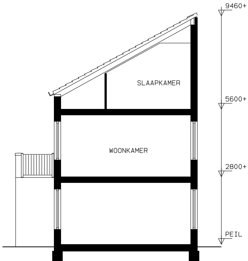
DOORSNEDE
