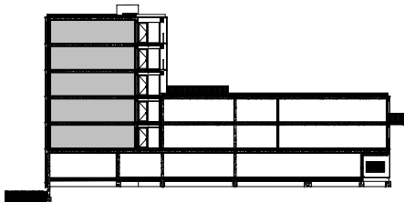
doorsnede A-A
