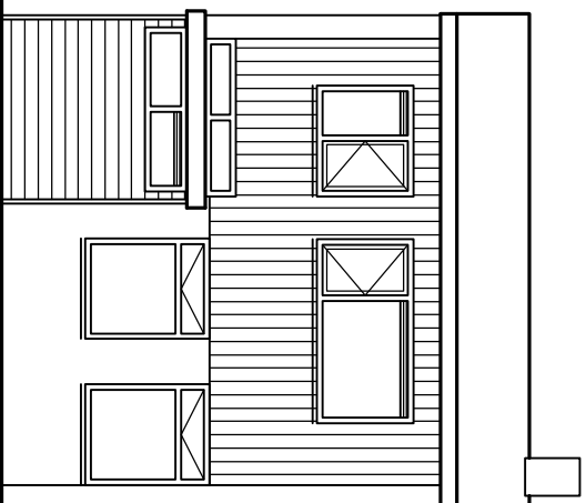
Achtergevel
