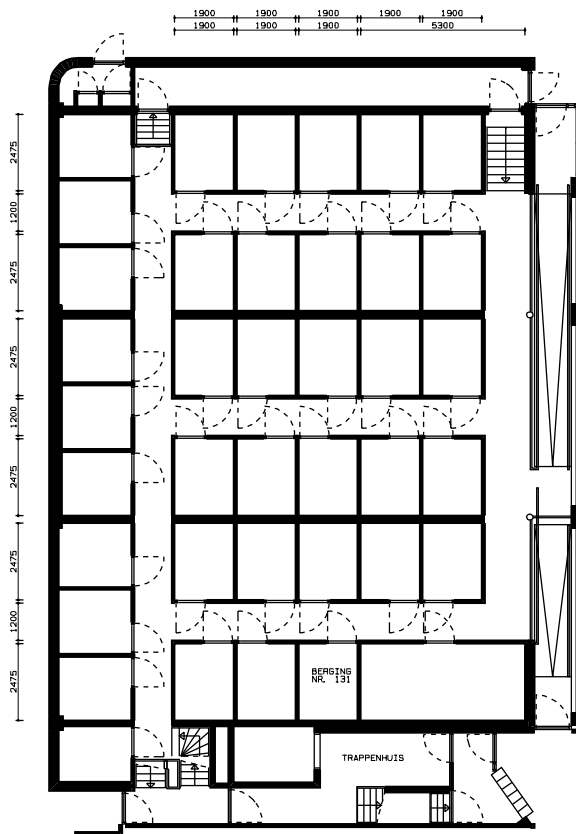
BEGANE GROND T. P. V. AAGJE DEKENPLEIN
