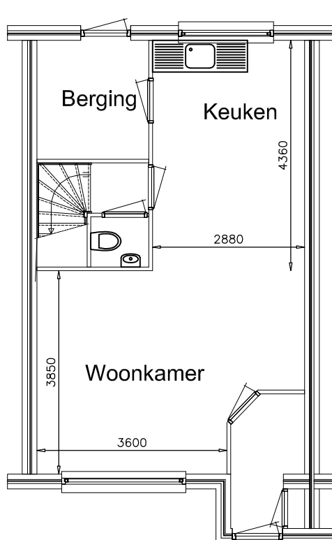
Begane grond
