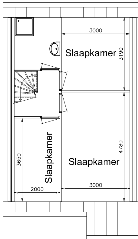
1e verdieping
