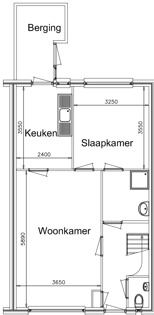
Begane grond
