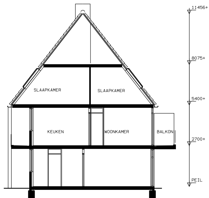
DOORSNEDE
