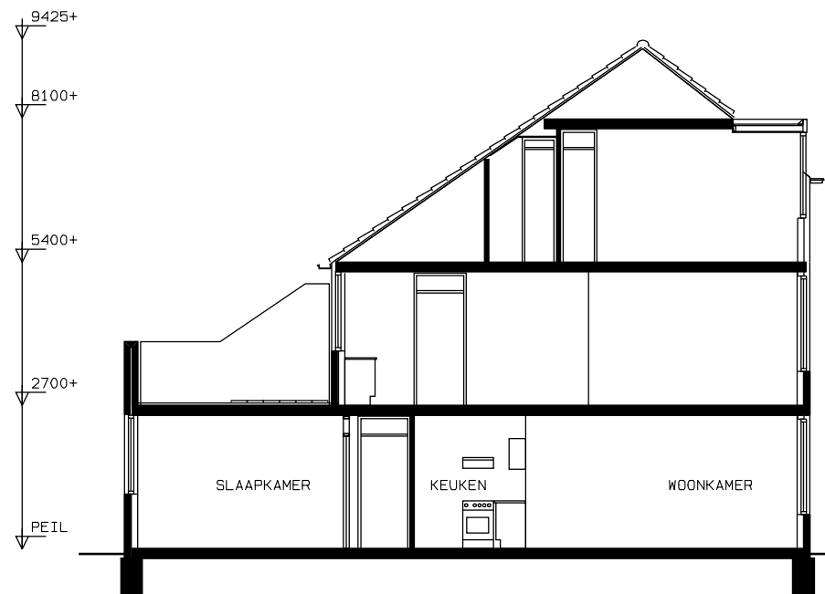
DOORSNEDE
