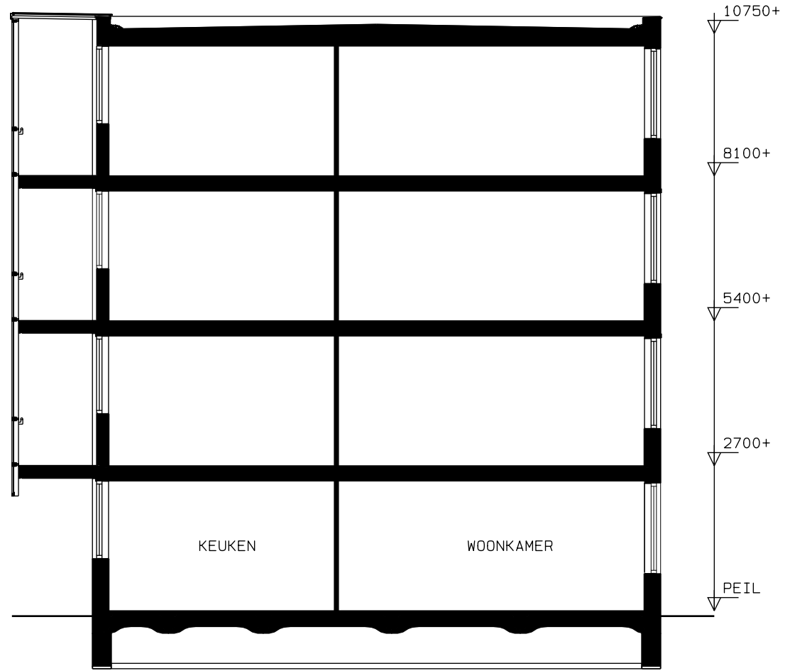
DOORSNEDE
