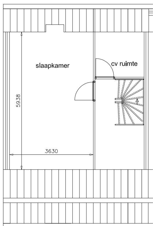
2e verdieping
