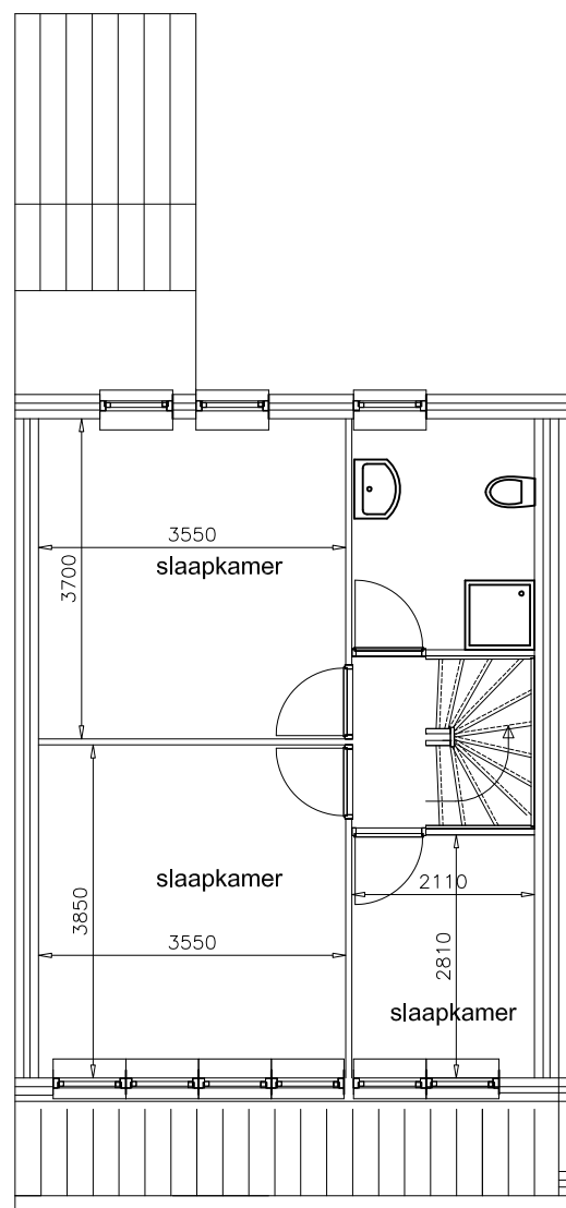
1e verdieping
