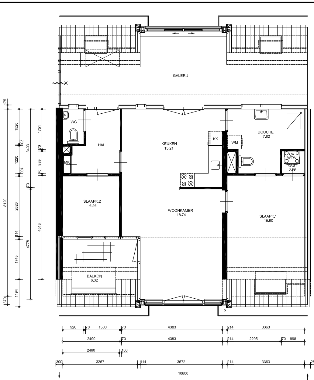
1E VERDIEPING
