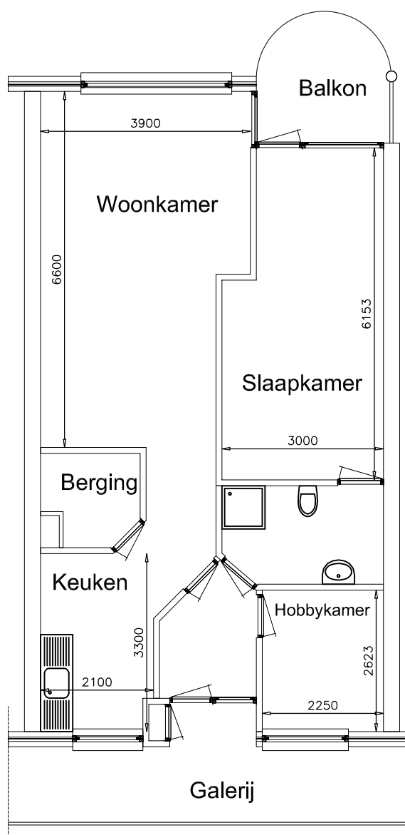
1e verdieping
