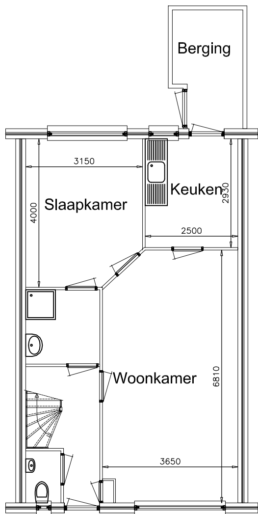
Begane grond
