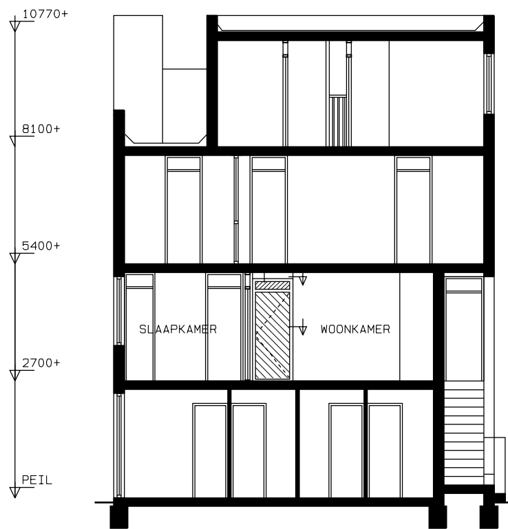
DOORSNEDE
