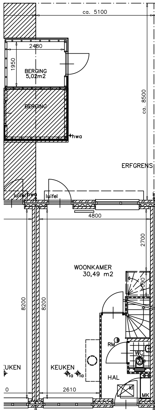
Begane grond
