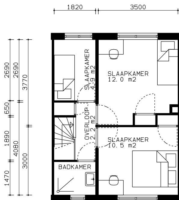
1e VERDIEPING
