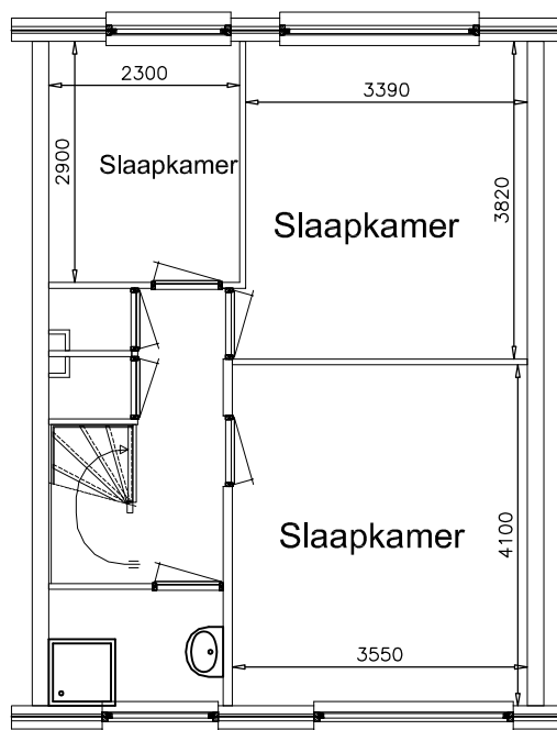
1e verdieping
