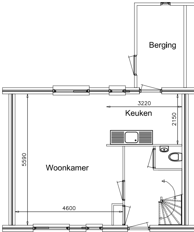
Begane grond
