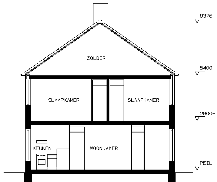
DOORSNEDE
