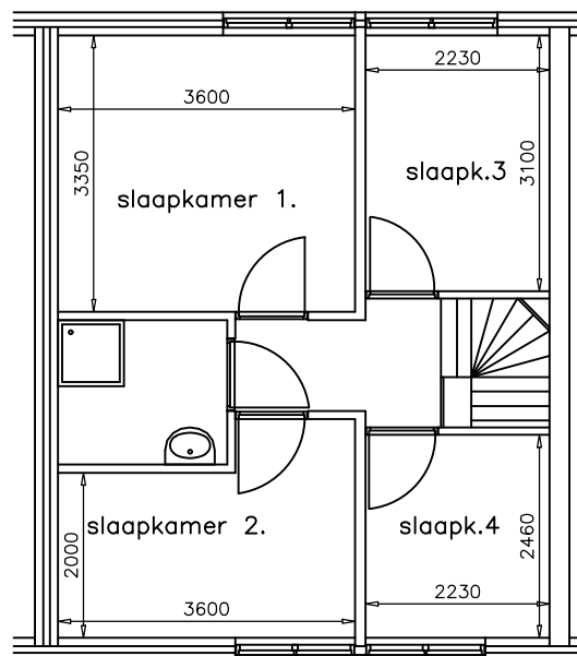
1e verdieping
