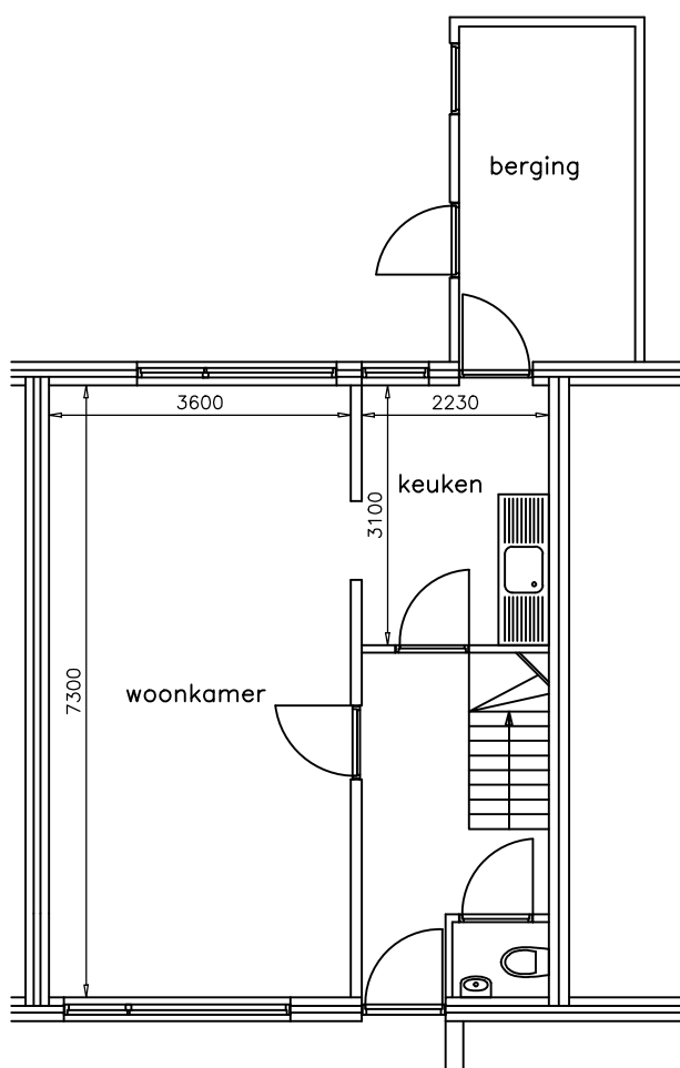
beganegrond
