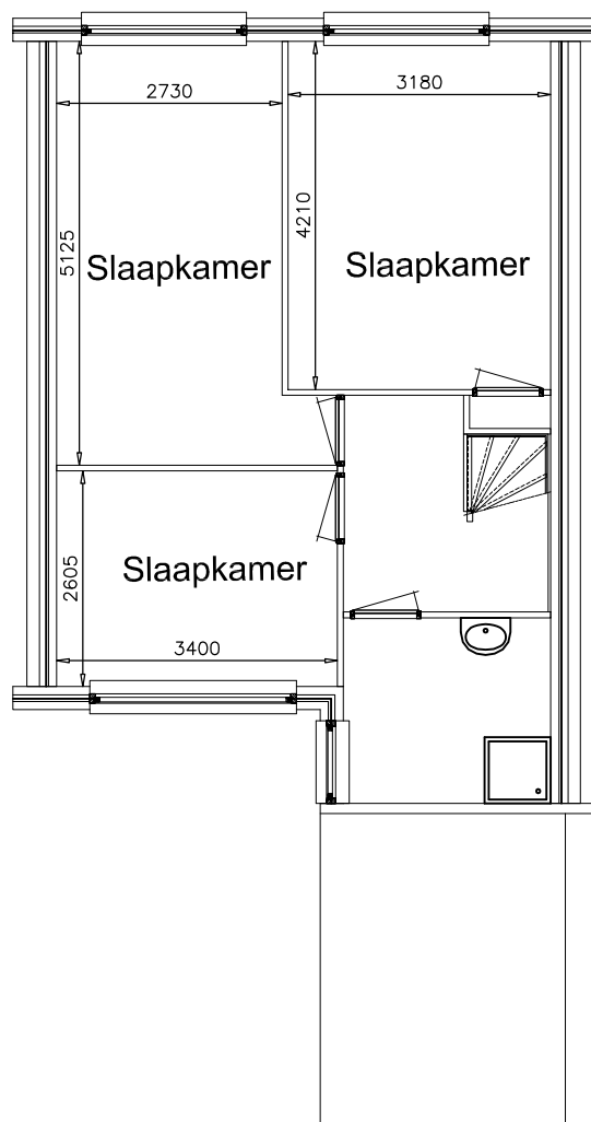
1e verdieping
